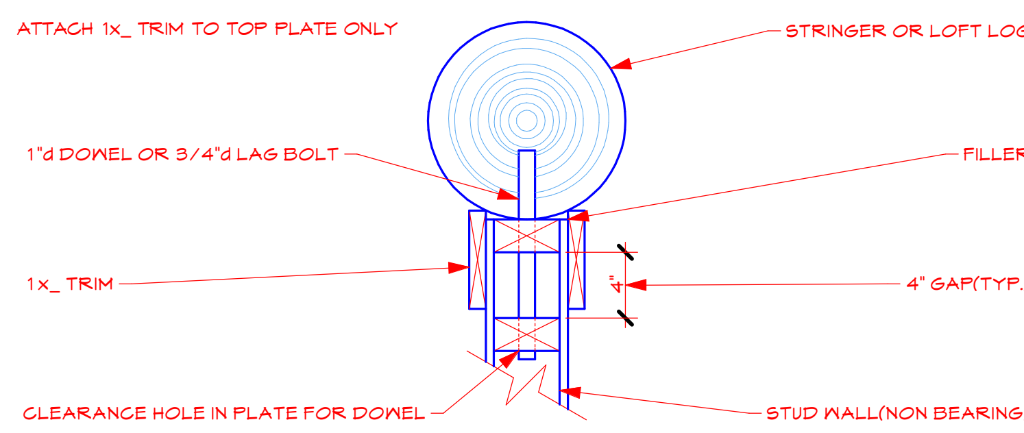
D25 SLIP JOINT DETAIL SCALE: 1 1/2" = 1'-0"
