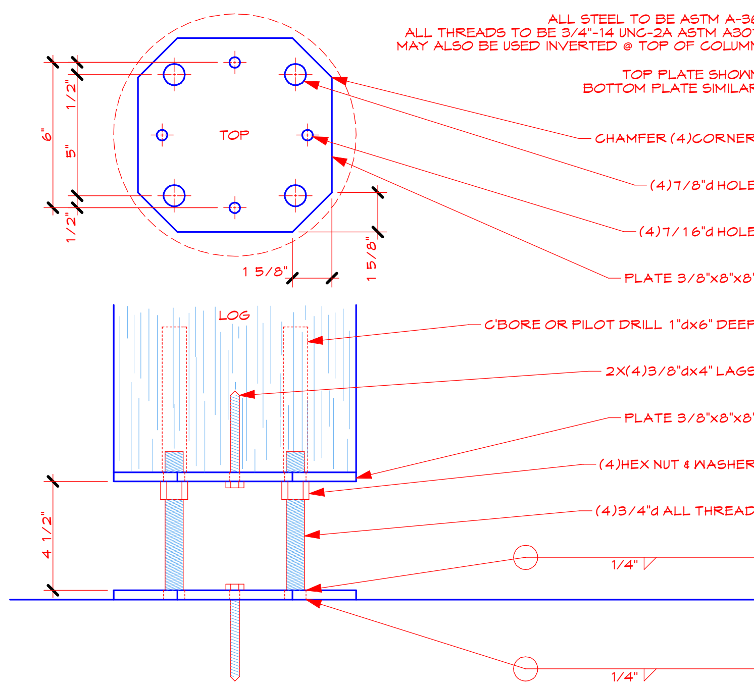
D24 TYPE 3 ADJUSTER DETAIL SCALE: 3/4" = 1'-0"
