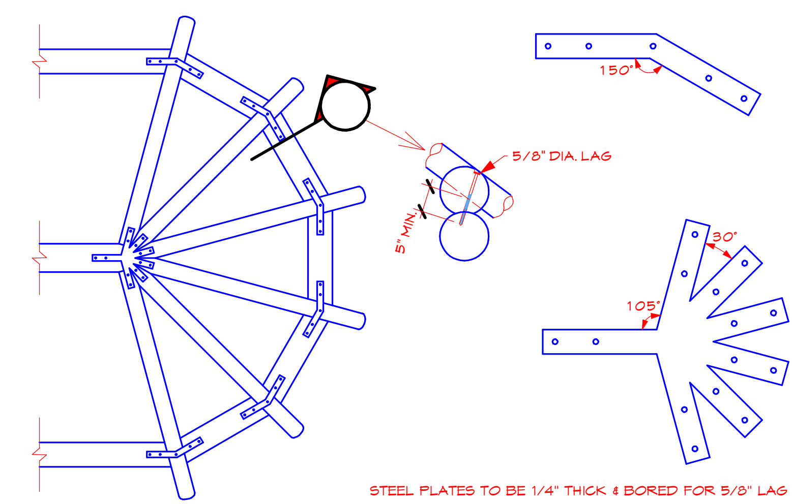
D32 LOG RAFTER CONNECTIONS N.T.S.
