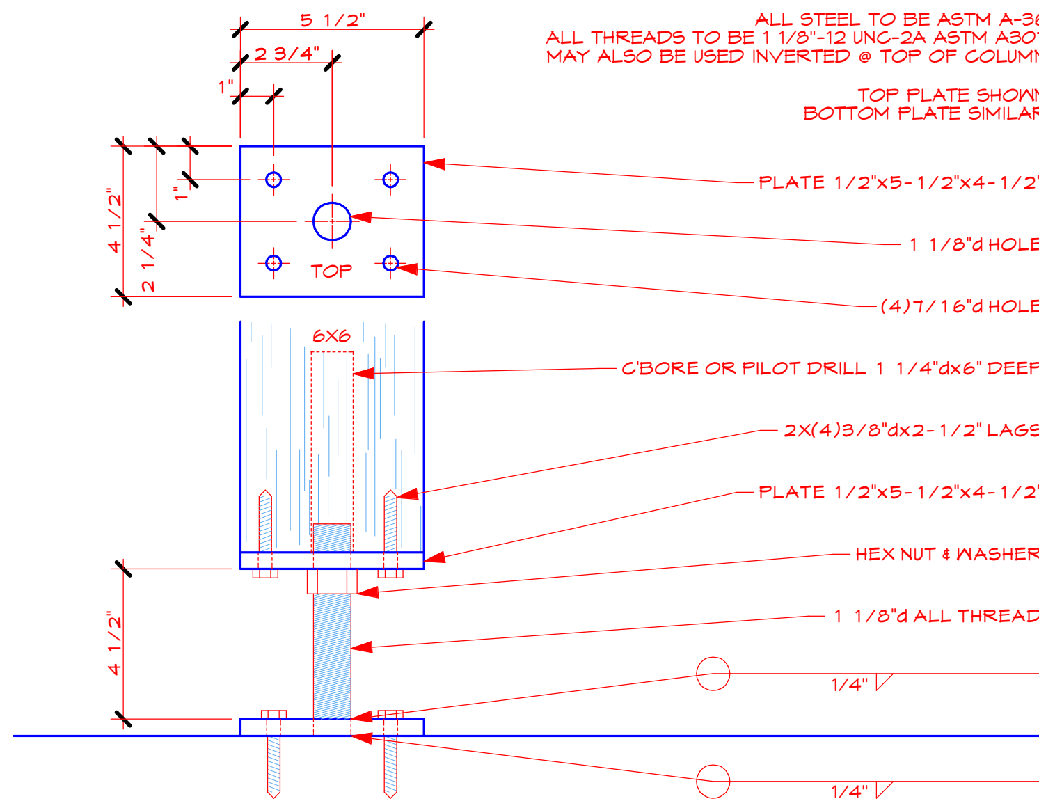
D23 TYPE 2 ADJUSTER DETAIL SCALE: 3/4" = 1'-0"
