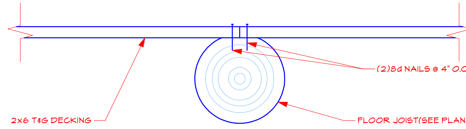
D26 LOFT LOG TO DECKING SCALE: 1 1/2" = 1'-0"
