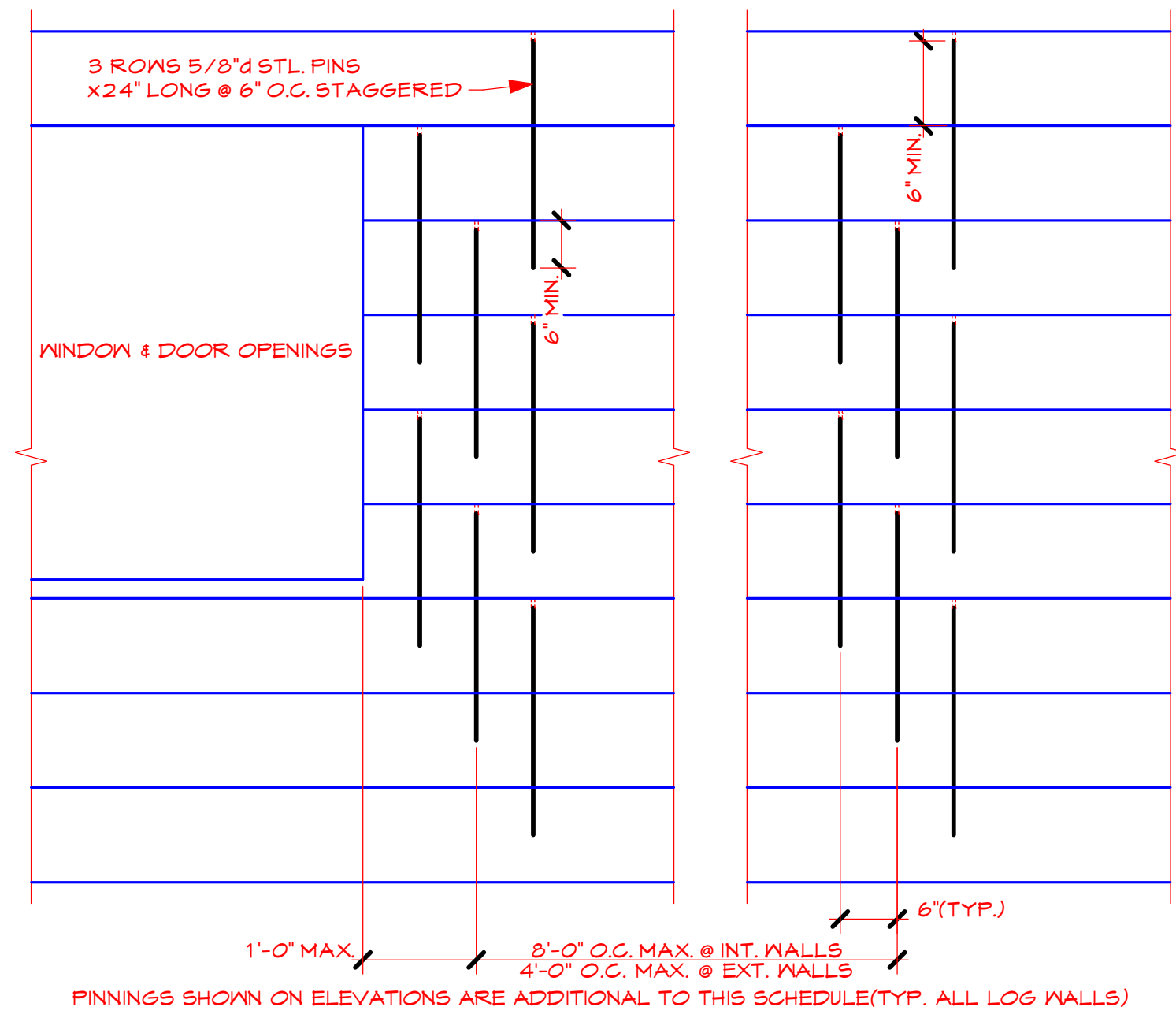
D22 PIN DETAIL SCALE: 3/4" = 1'-0"
